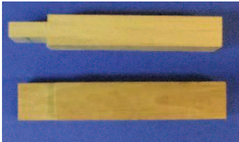
15. Winkelärmchen, roh, mit Zapfen Weißbuche, 65 x 12 x 9
