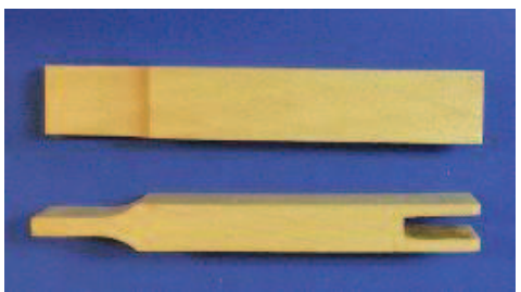
17. Winkelärmchen, roh Weißbuche, 65 x 12 x 7
